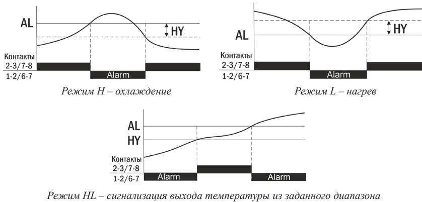
Рис. 2 – Режимы работы
