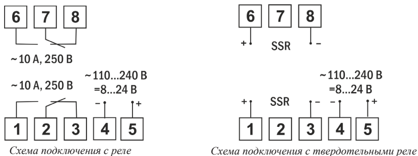
Рис. 3 – Схемы подключения
